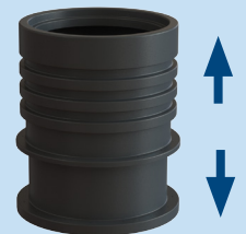
CPX Teleskophals Diameter / Höjd 600 mm / Justerbar 600-1000 mm Installationsdjup 600 – 1000 mm Passar till Cipax tankar
